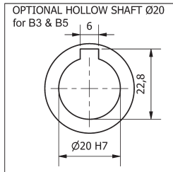
OPTIONAL HOLLOW SHAFT Ø20 for B3 & B5
